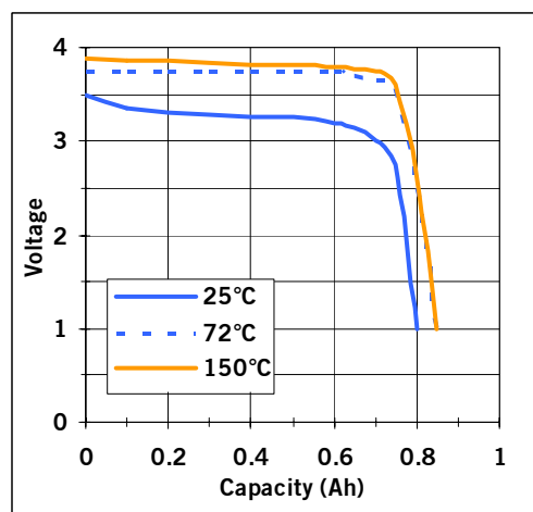
20 mA discharge
