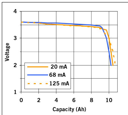
150°C discharge
