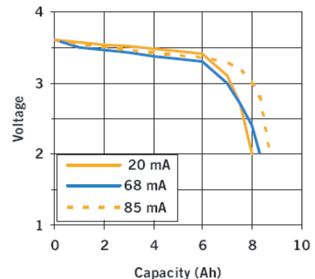
150°C discharge
